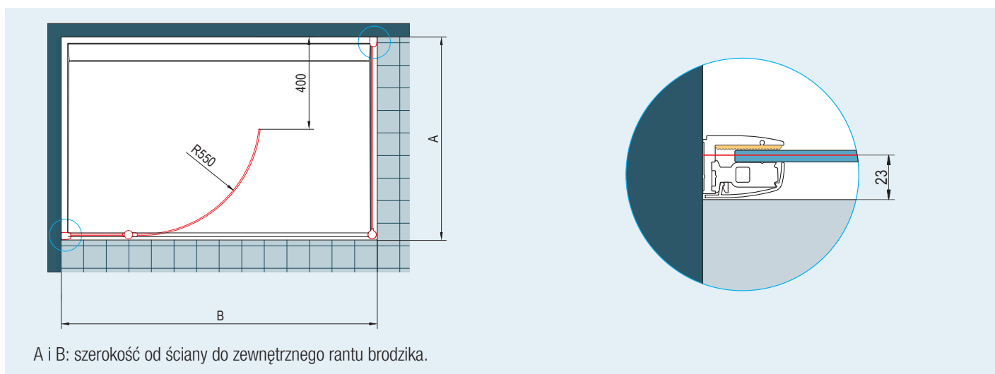
Widok 2: Przesunięcie sztyby do wewnątrz od zewnętrznego rantu brodzika o 23 mm jest stałe przy wszystkich modelach z serii Salsa
